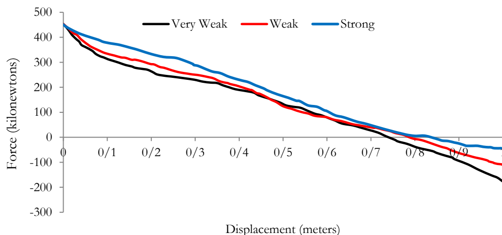
Fig. 13. Force-versus-displacement diagram.
